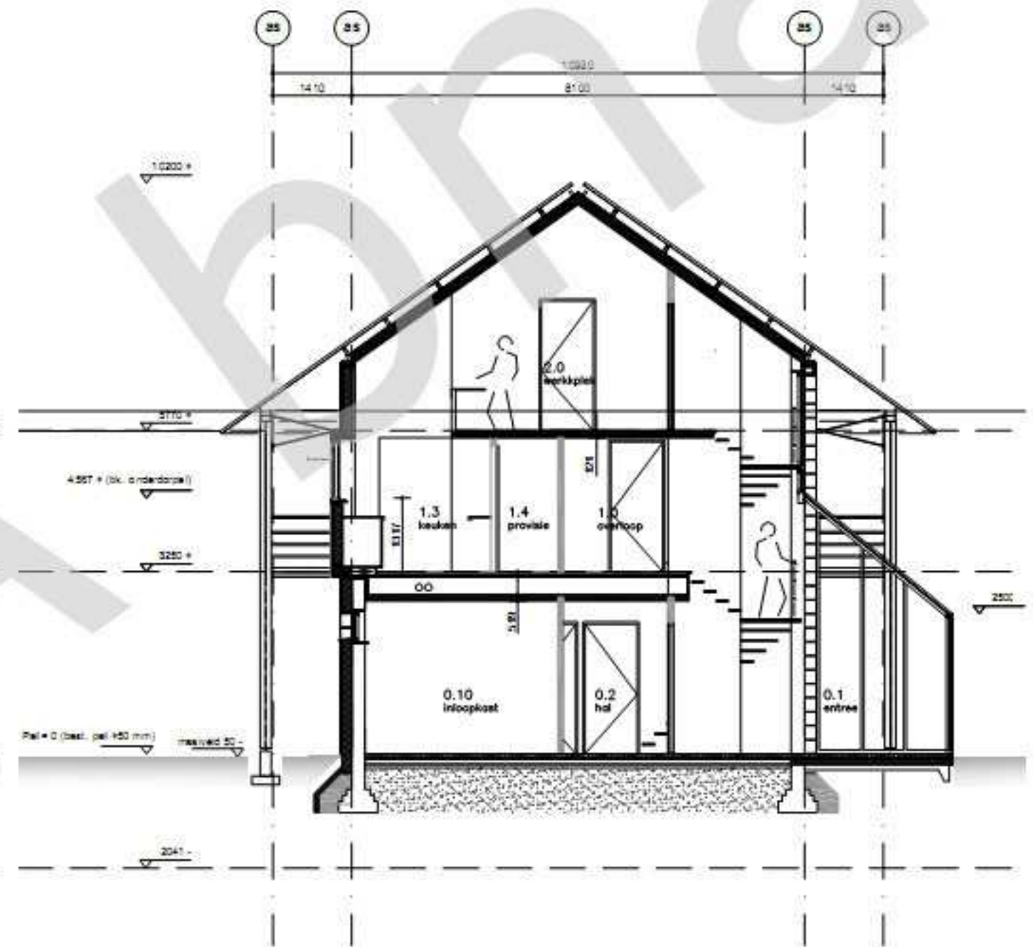
doorsnede B-B
