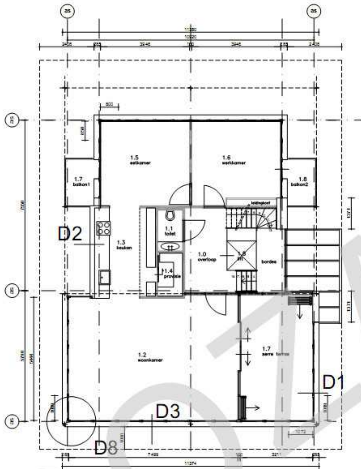
1e verdieping
