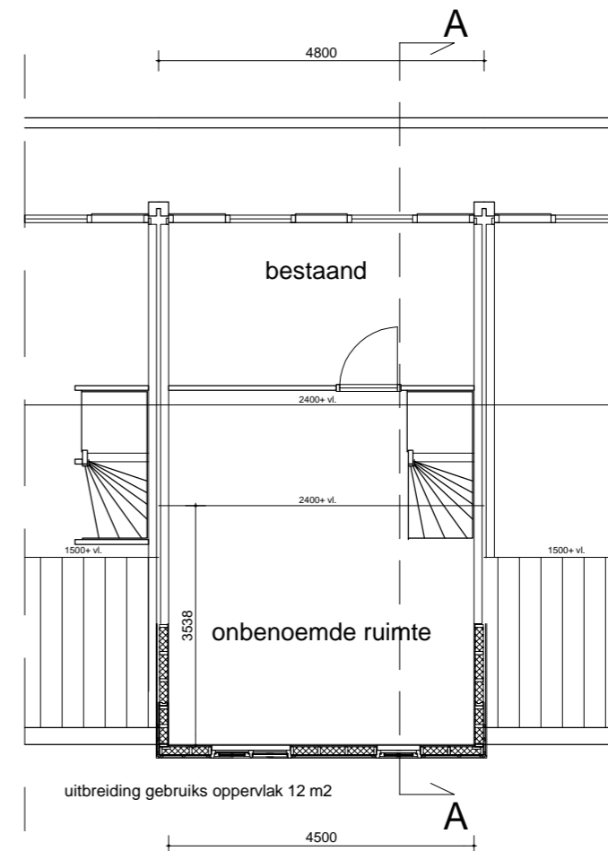
2e verdieping
