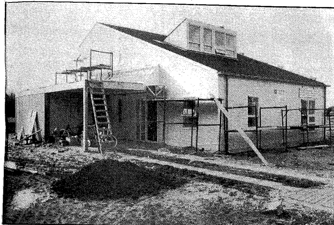
De woning aan Houtvester in de nieuwe wijk Bosveld. Behalve de vorm wijkt de woning ook af door het ontbreken van bakstenen. Het uiterlijk van het huis wordt nu nog overheerst door de blokken polyurethaanschuim (wandisolatie) die afgewerkt zullen worden met stukwerk dat geschilderd kan worden.
